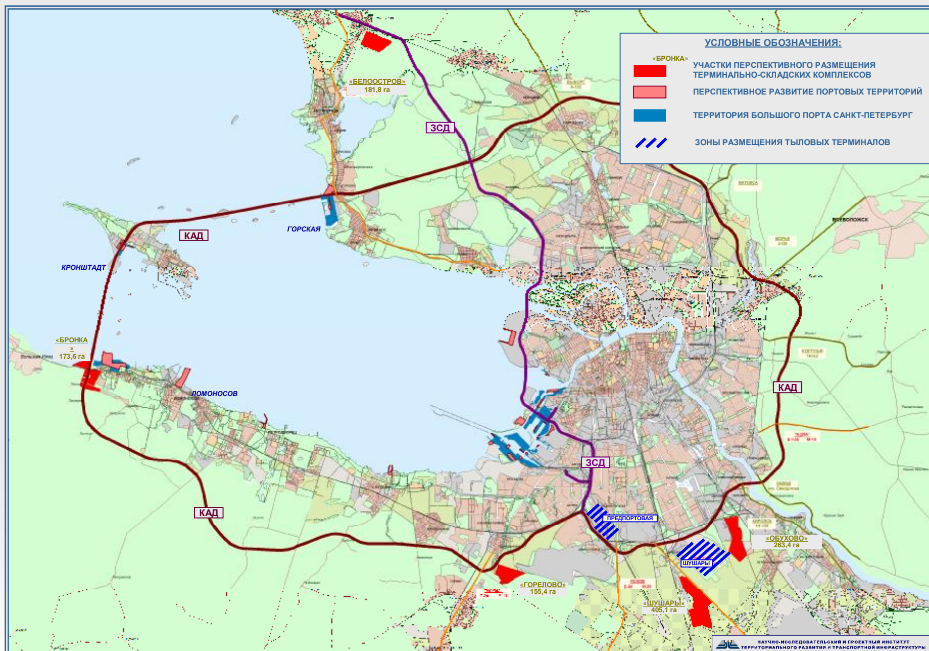
СХЕМА ПЕРСПЕКТИВНОГО РАЗМЕЩЕНИЯ ПОРТОВЫХ ТЕРРИТОРИЙ И КРУПНЕЙШИХ ЛОГИСТИЧЕСКИХ ТЕРМИНАЛОВ В САНКТ-ПЕТЕРБУРГЕ
