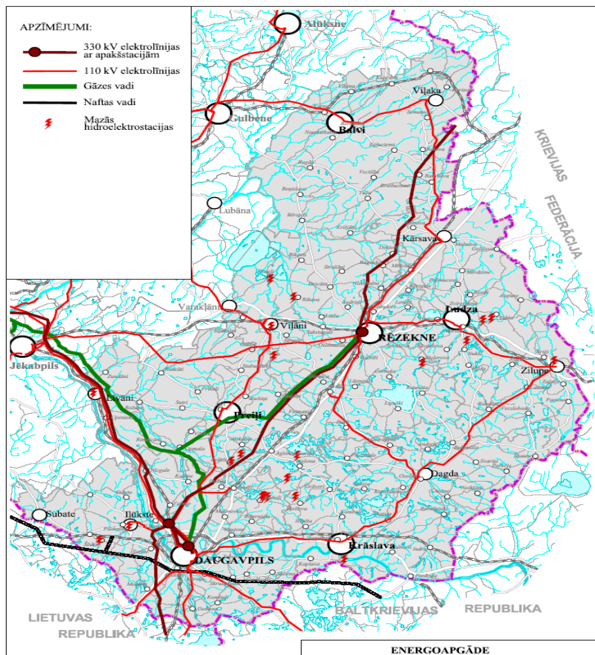
25. attēls Energoapgāde Latgales reģionā
