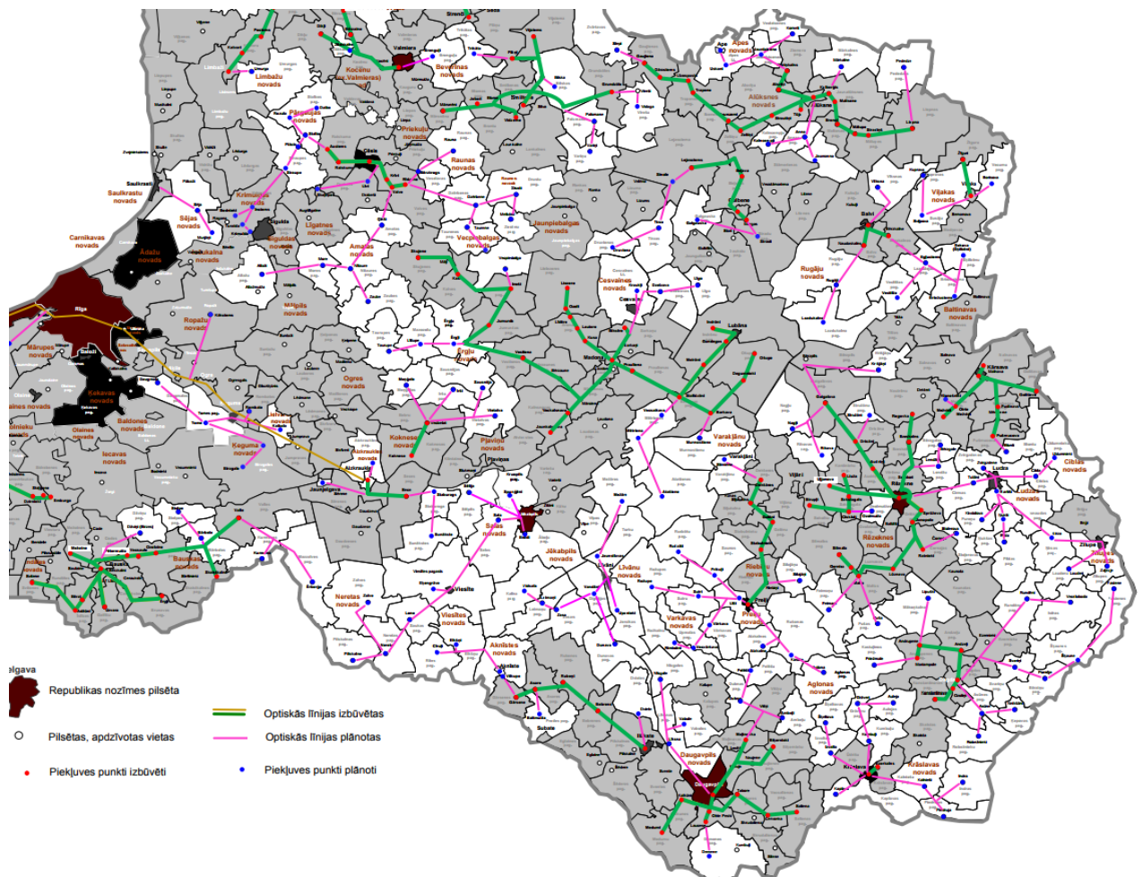
28.attēls Platjoslas interneta tīkls (zaļš – I kārta, rozā – II kārta)
